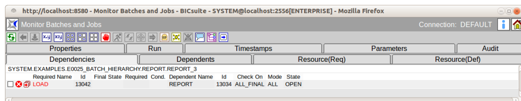
Figure 22.12: Batch und job dependencies
