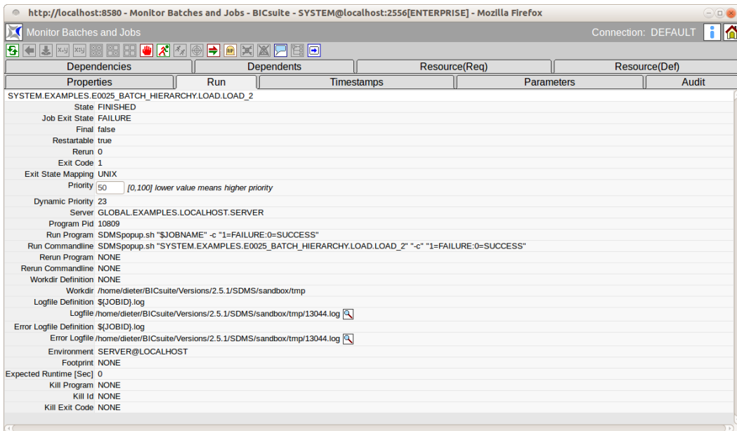
Figure 22.10: Batch und Job Run information
